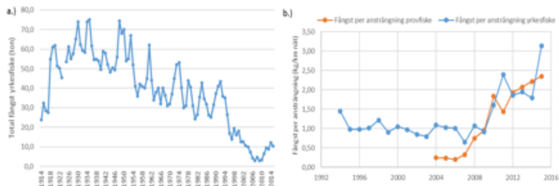
Figur 10. a) Totala fångster av röding (ton) från yrkesfisket 1914-2015 och b) fångster av röding per ansträngning (kg/km nät) i provfiske 2004-2015 (orange linje) och i yrkesfisket 1994-2015 (blå linje).
